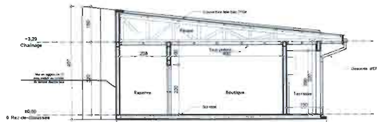
COUPE A-A
